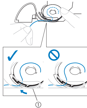
1 Пружина регулировки натяжения нити
